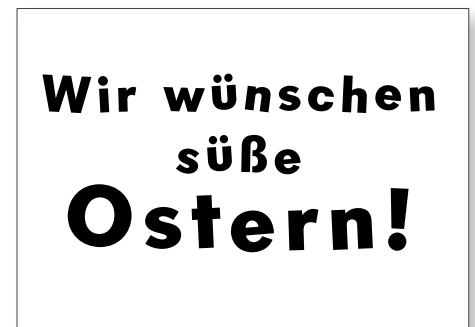
SO3
